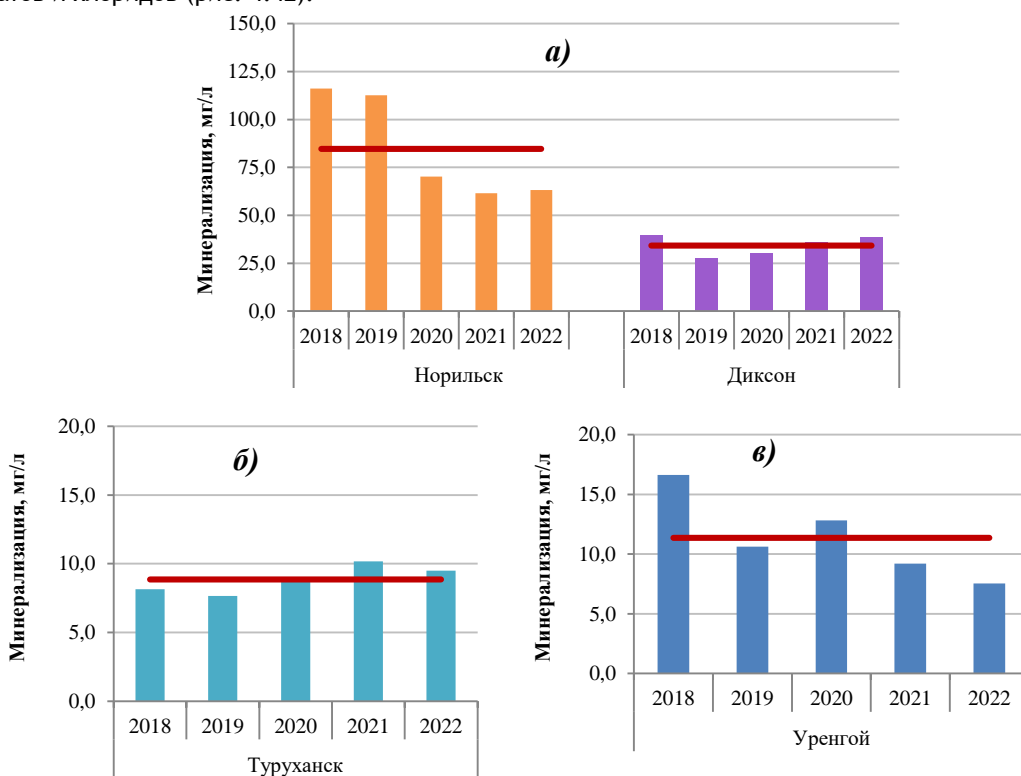
Рис. 4.41. Изменение средневзвешенной минерализации осадков на территориях Красноярского края (а, б) и Ямало-Ненецкого АО (в), 2018-2022 гг.
