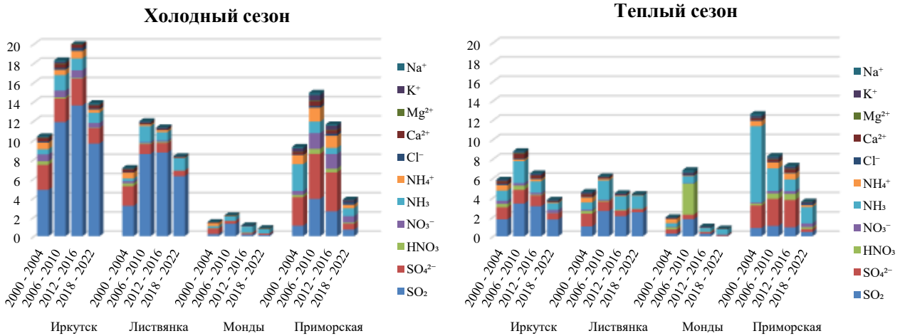
Рис. 2.39. Изменение средних пятилетних значений содержания кислотообразующих веществ в общем составе аэрозолей и газов (мкг м -3 ) на станциях ЕАНЕТ в холодный (слева) и теплый (справа) периоды в 2000-2022 гг.
