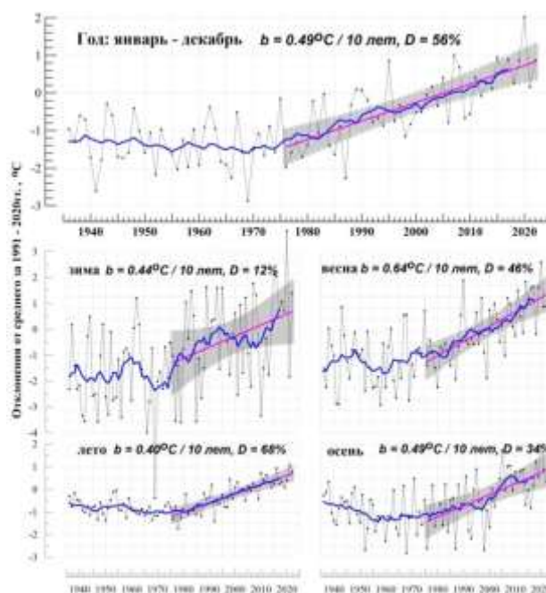
Рис. 1.8. Средние годовые (вверху) и сезонные аномалии температуры приземного воздуха (°C), осредненные по территории РФ, 1936-2022 гг.
