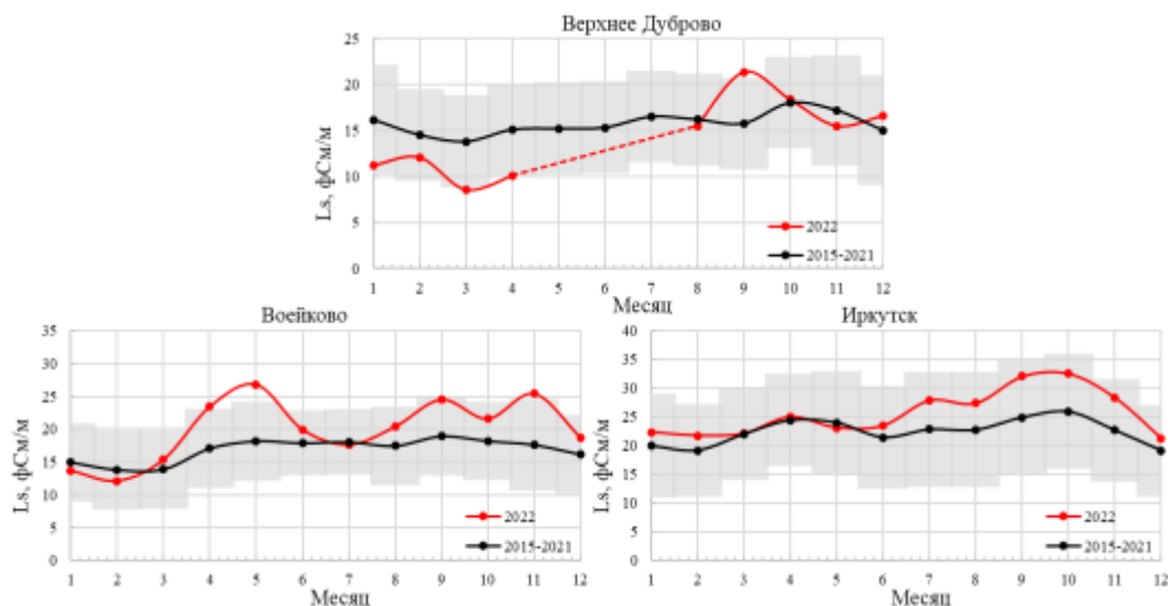
Рис. 2.10. Годовой ход L_5 на станциях Верхнее Дуброво, Воейково, Иркутск в 2022 г. на фоне осредненного годового хода L_5 за период 2015-2021 гг.
