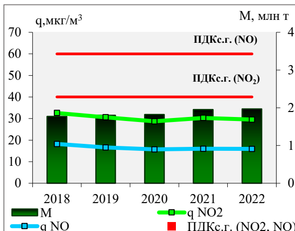
Рис. 3.12. Среднегодовые концентрации диоксида азота (qNO₂, мкг/м³) и оксида азота (qNO, мкг/м³) и выбросы от стационарных источников (M, млн т) NOx (в пересчете на NO₂)
