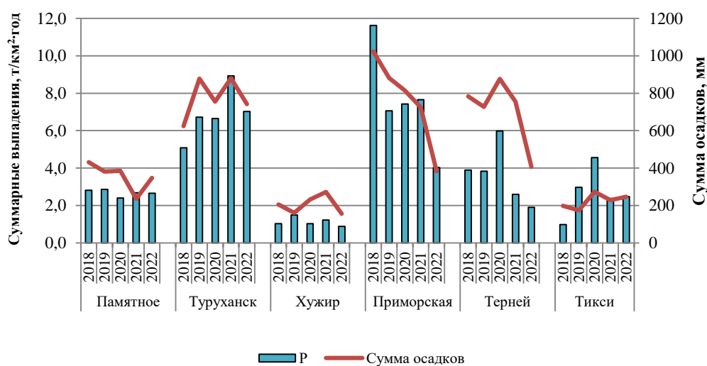
Рис. 2.24. Суммарные влажные выпадения на АЧР, 2018-2022 гг.
