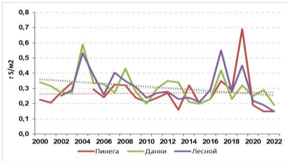
Рис. 2.36. Многолетние выпадения сульфатной серы из атмосферы с осадками на станциях ЕМЕП (г S/m 2 /год)
