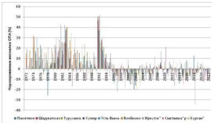
Рис. 2.8. Нормированные аномалии ОПА(%) на станциях фоновый мониторинга
