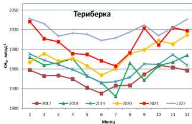
Рис. 2.2. Сезонный ход концентрации CH 4 на станции Териберка
