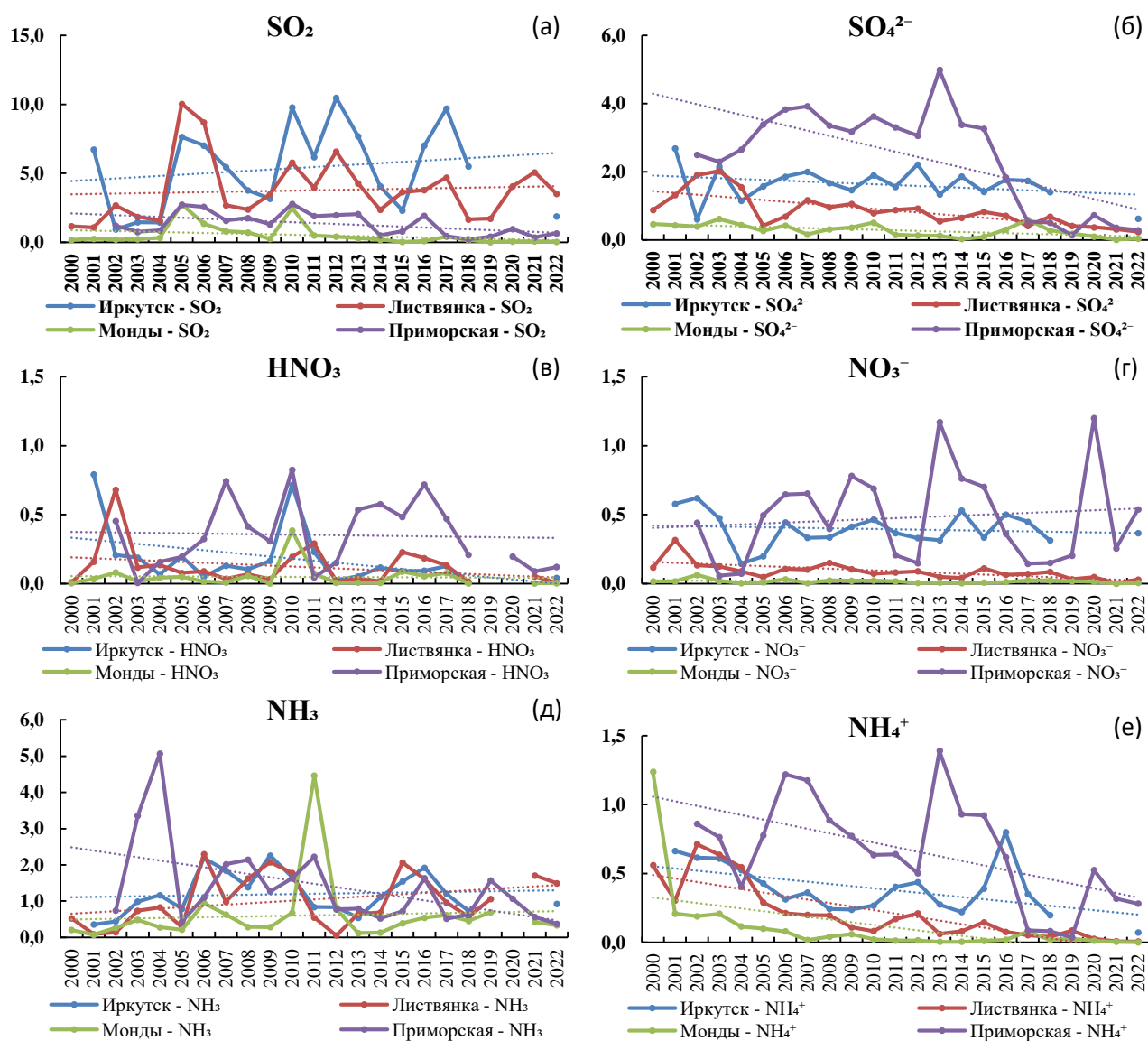
Рис. 2.38. Изменения средних годовых концентрации соединений серы (а, б) и азота (в, г, д, е) в атмосферном воздухе на станциях ЕАНЕТ ( \mu\text{кг м}^{-3} )
