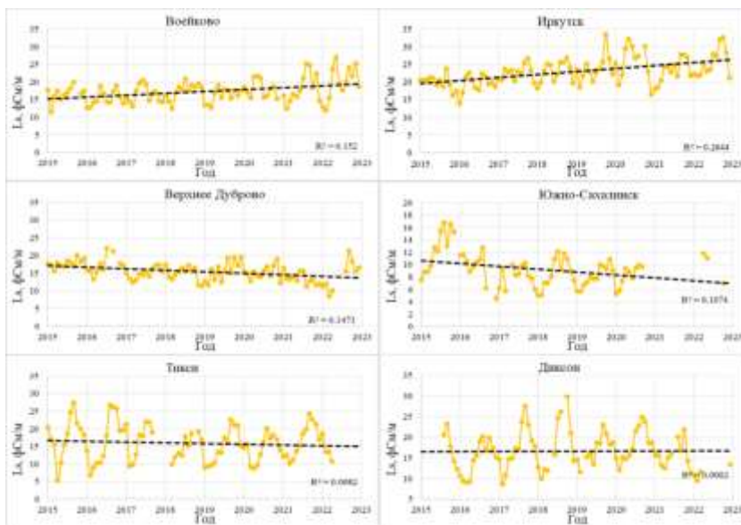
Рис. 2.12. Среднемесячные тренды Ls на сети станций мониторинга ЭХА
