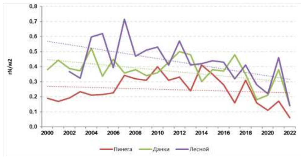
Рис. 2.37. Многолетние выпадения суммарного азота (нитратного и аммонийного) из атмосферы с осадками на станциях ЕМЕП (г N/m 2 /год)
