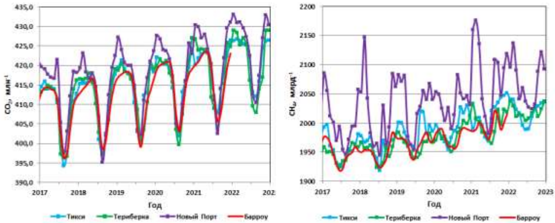
Рис. 2.1. Временной ход концентрации CO 2 и CH 4 на российских арктических станциях в сравнении с данными станции Барроу
