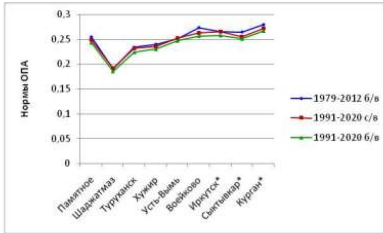
Рис. 2.6. 30-летние нормы ОПА, рассчитанные для каждой станции фоновый мониторинга за 1979-2012 гг. (без учета 1983-1984 гг.) и 1992-1993 гг. (6/в); за 1991-2020 гг. (полностью (с/в) и за 1991-2020 гг. (без учета 1983-1984 гг.) и 1992-1993 гг. (6/в)
