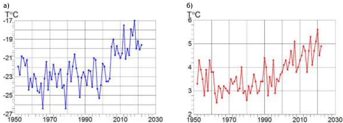
Рис. 4.35. Приповерхностная температура воздуха зимой (а) и летом (б) на акватории морей Северного морского пути
