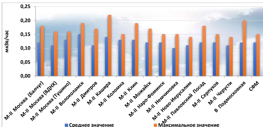
Рис. 4.8. Мощность AMBIENTНОГО эквивалента дозы гамма-излучения (МАЭД) в 2022 г.
