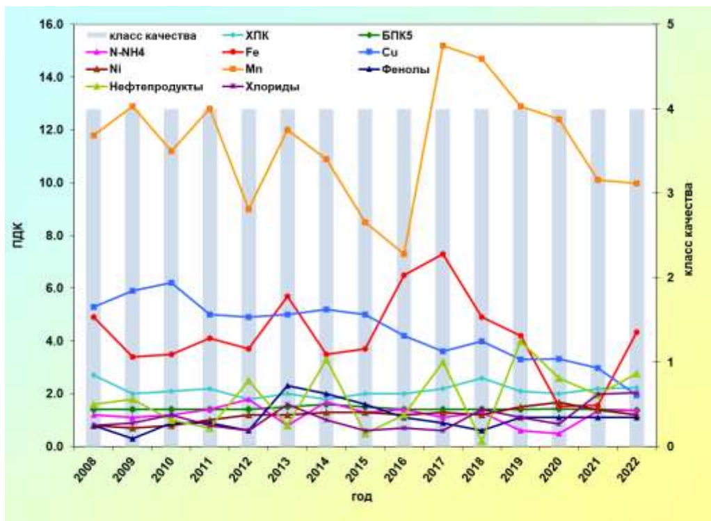
Рис 3.39. Изменение среднегодовых концентраций отдельных загрязняющих веществ и показателей качества воды р. Белая, 10,5 км ниже г. Стерлитамак за многолетний период
