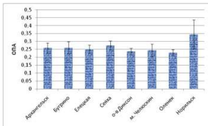
Рис. 4.39. Осредненные за наблюдательный период 2022 г. значения ОПА и их стандартные отклонения ( \pm ) на арктических станциях
